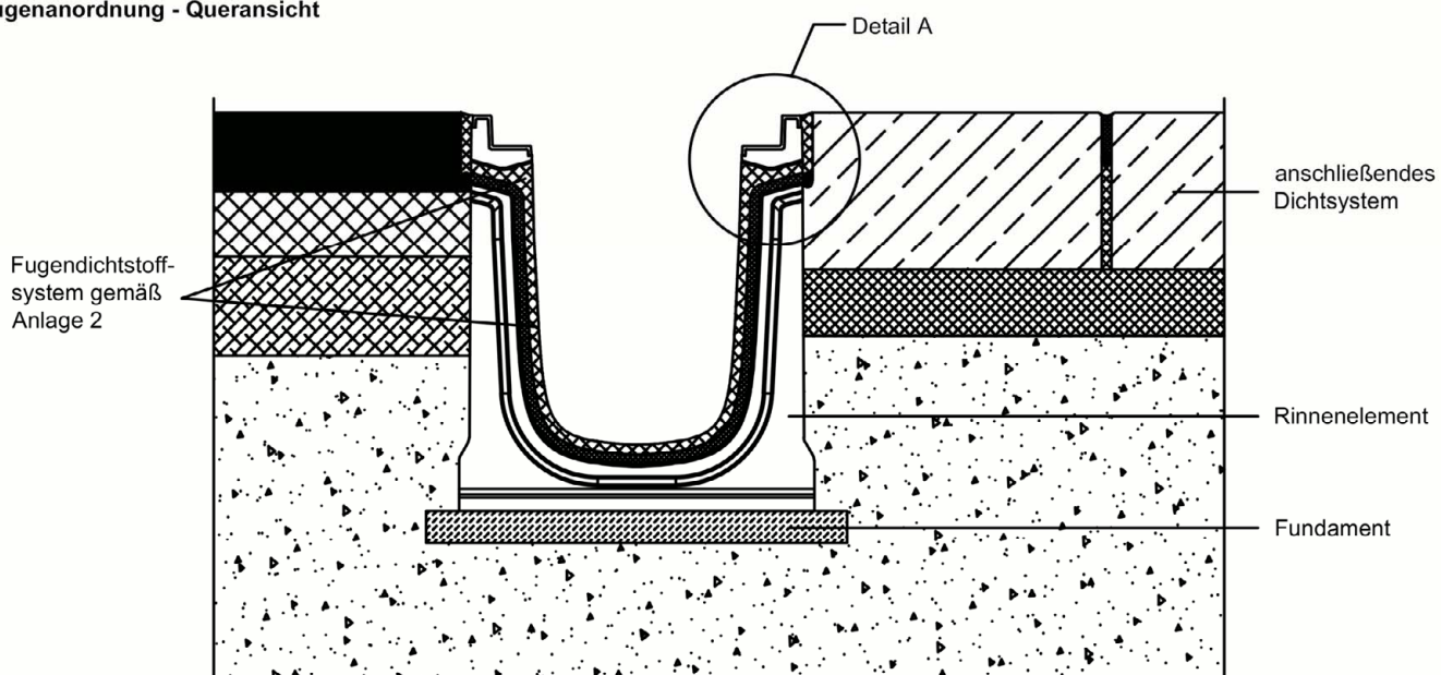
Fugenanordnung - Queransicht
