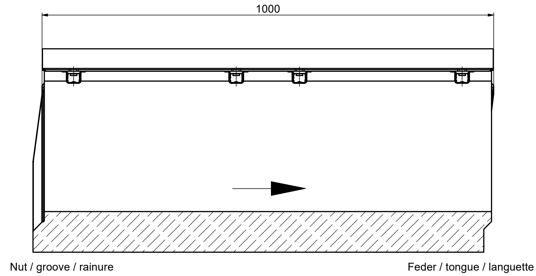
Schnitt / section / coupe A-A
