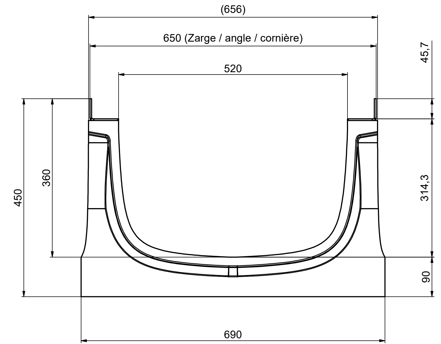
Ansicht Nut / view groove / vue rainure
