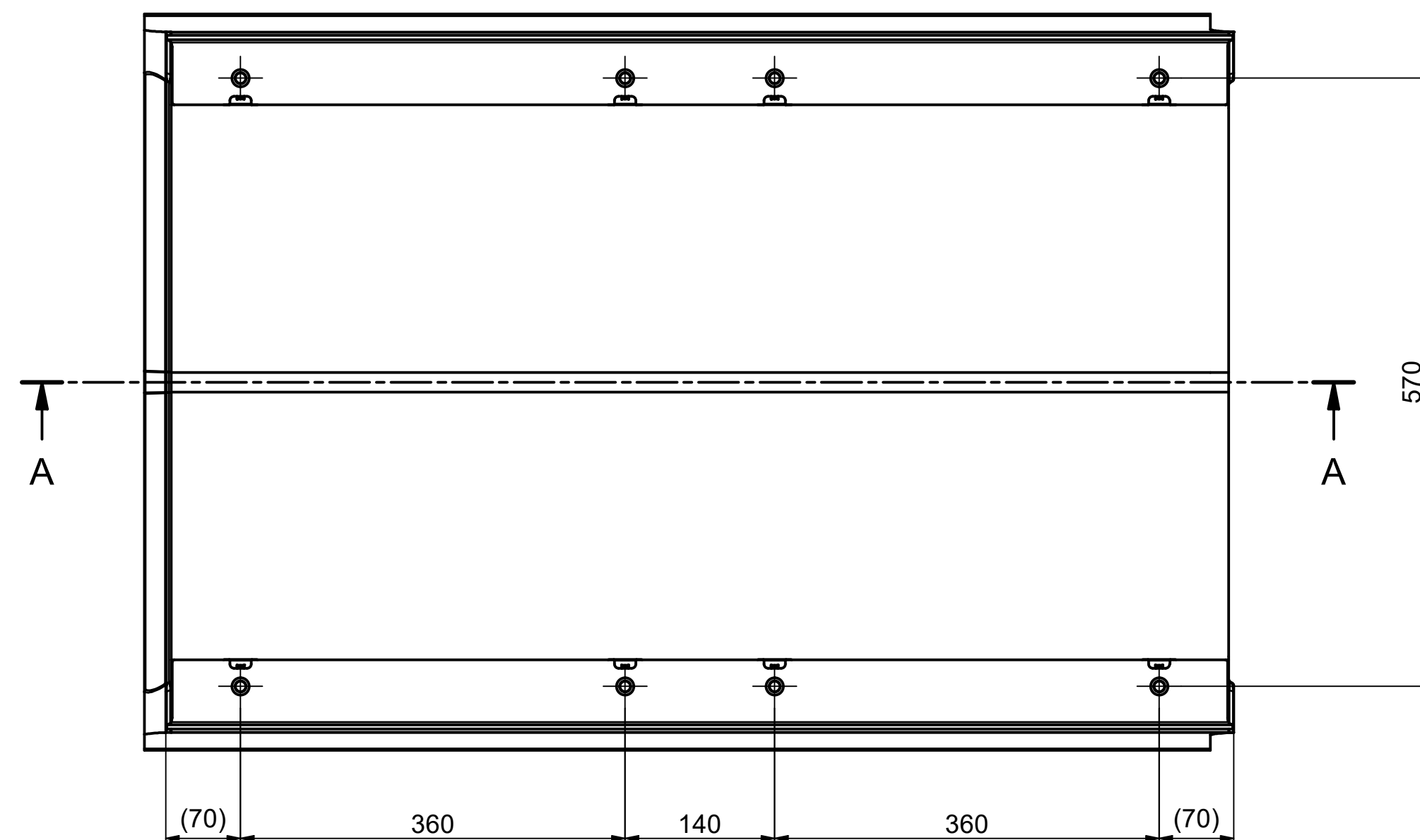
Draufsicht / top view / vue de dessus
