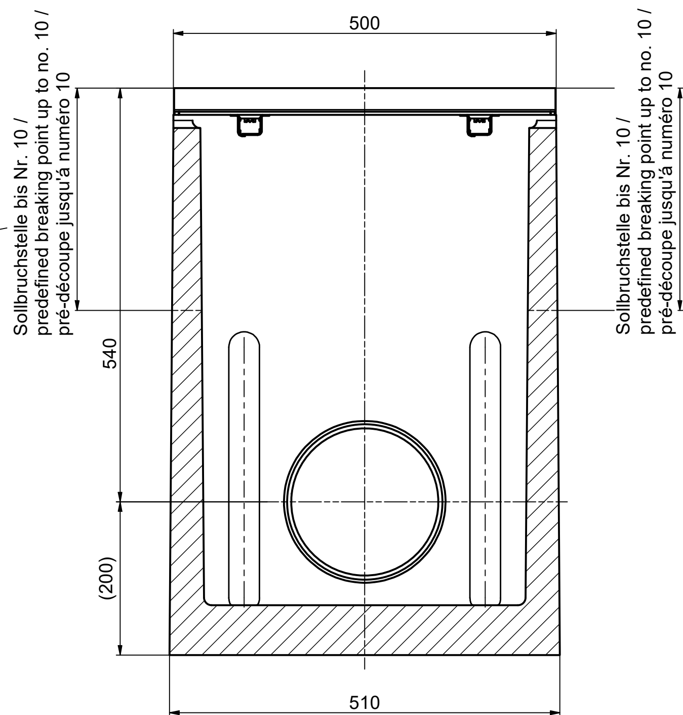
Schnitt / section / coupe B-B
