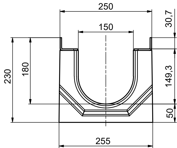
Ansicht Feder / view tongue / vue languette
