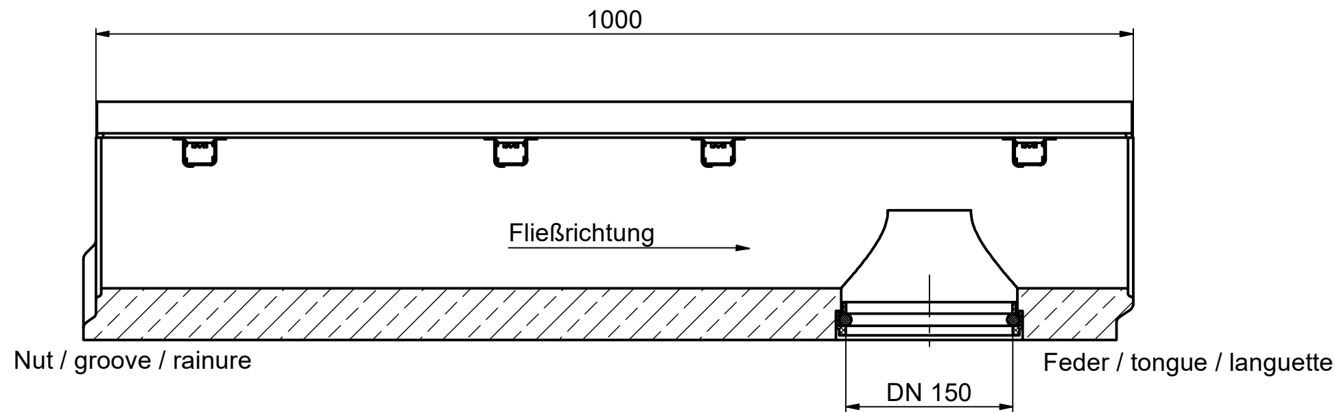
Schnitt / section / coupe A-A
