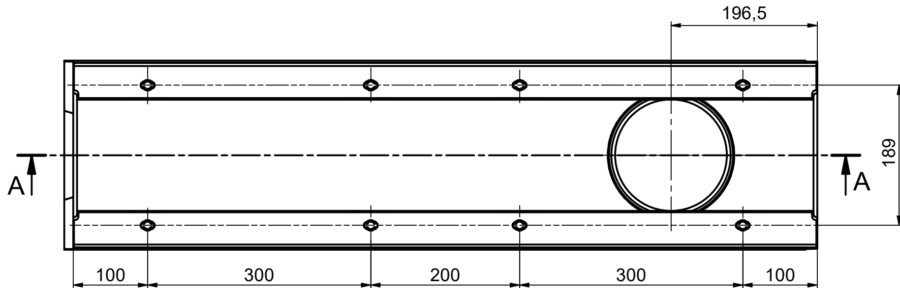
Draufsicht / top view / vue de dessus
