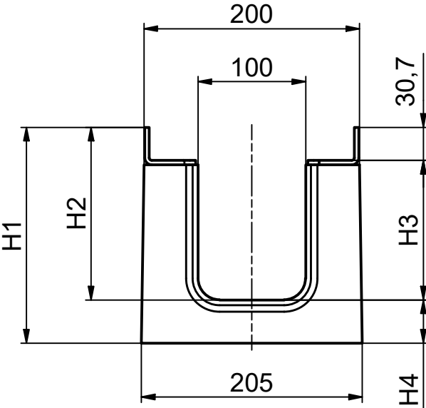
Seitenansicht / side view / vue de côté
