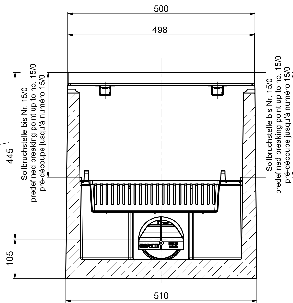
Schnitt / section / coupe B-B
