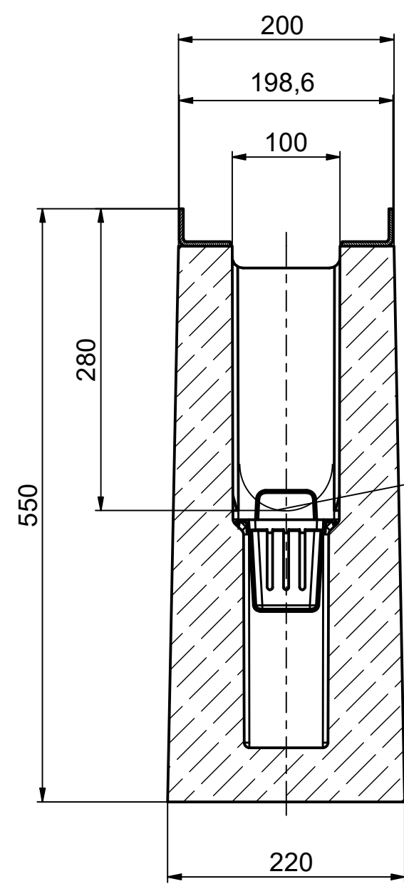
Schnitt / section / coupe A-A
