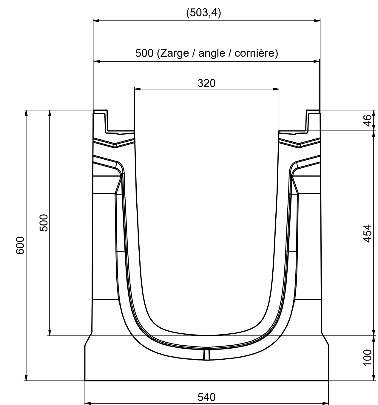
Ansicht Nut / view groove / vue rainure
