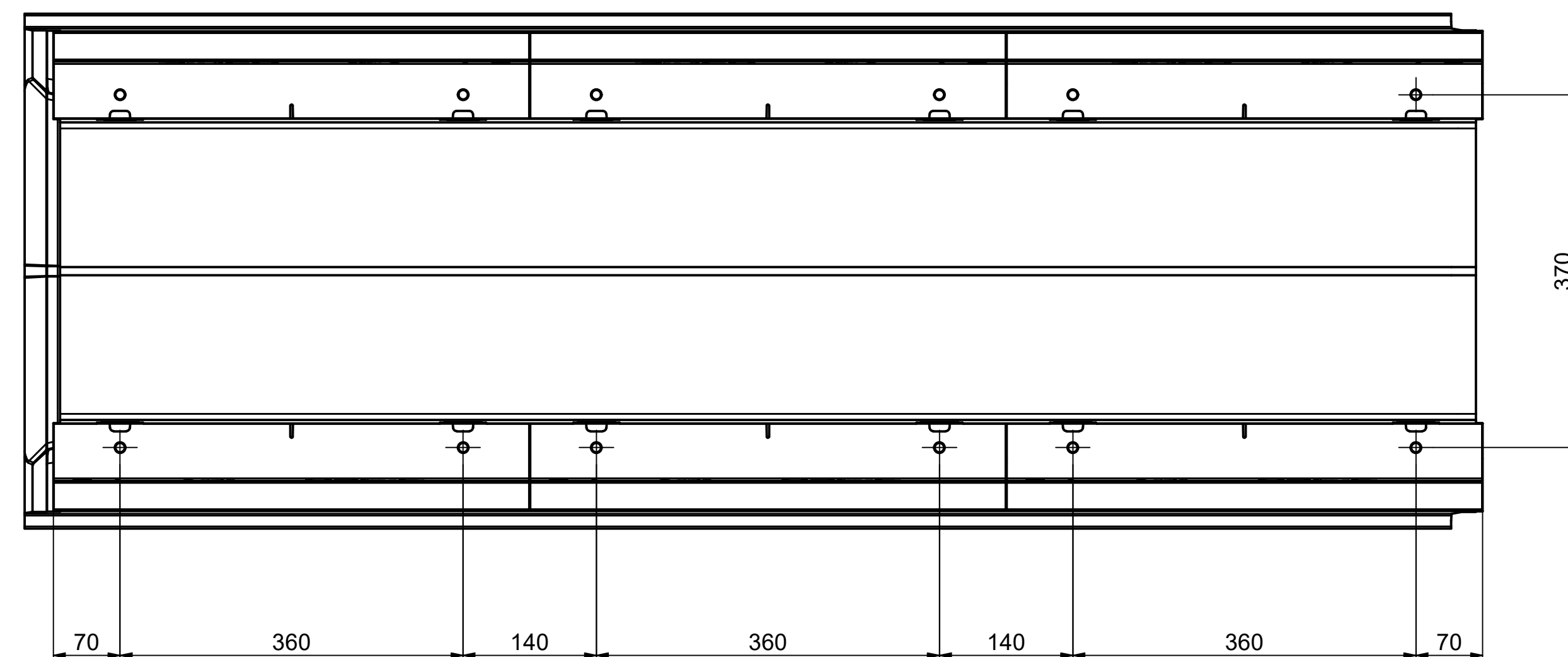
Draufsicht / top view / vue de dessus
