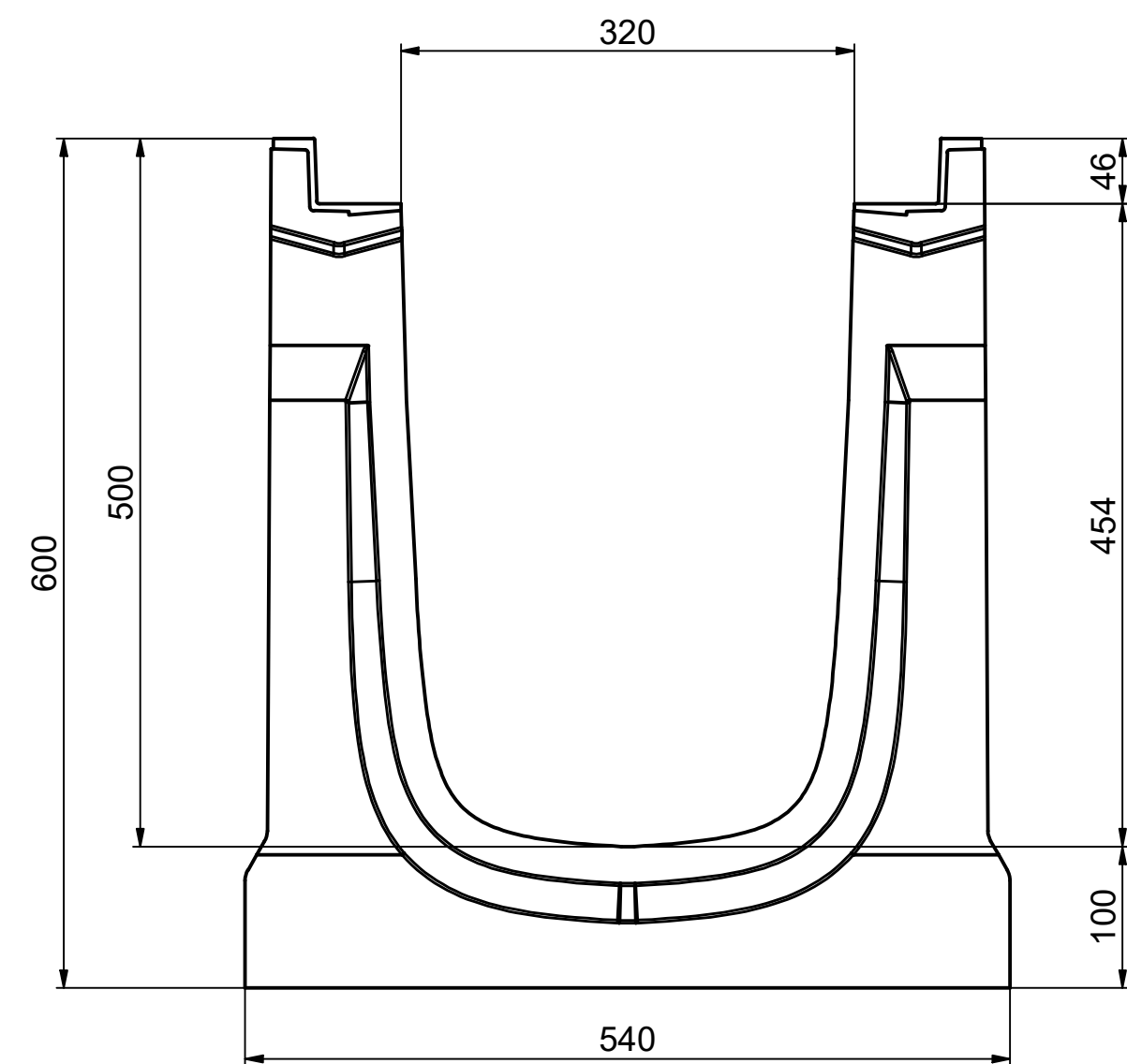
Ansicht Feder / view tongue / vue languette
