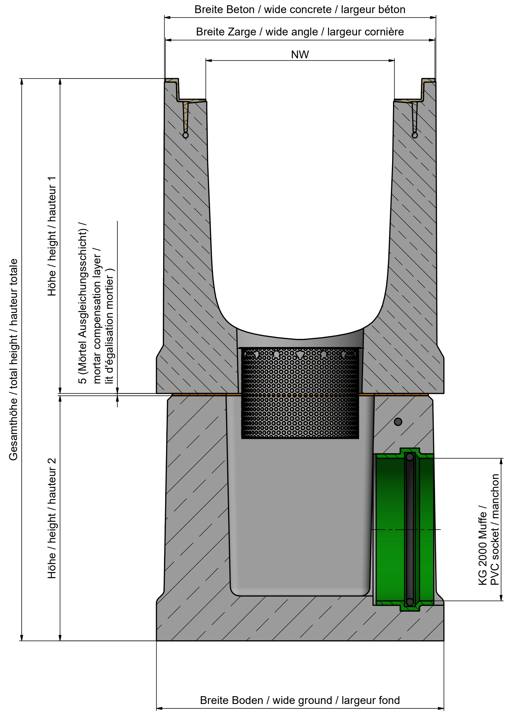
Schnitt / section / coupe B-B
