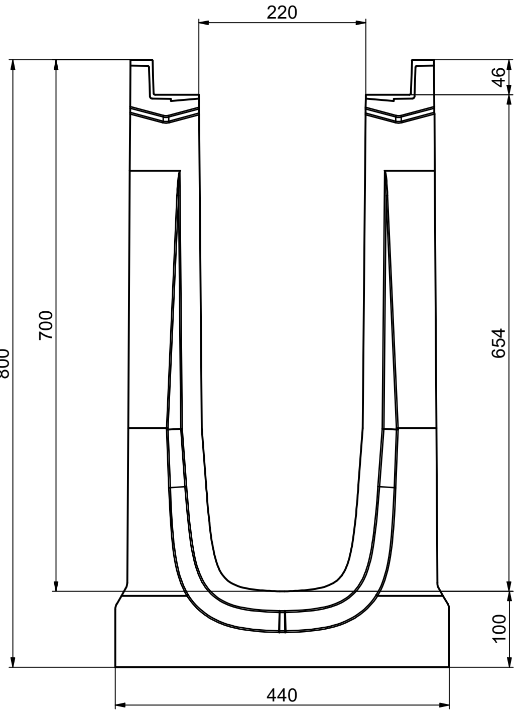
Ansicht Feder / view tongue / vue languette
