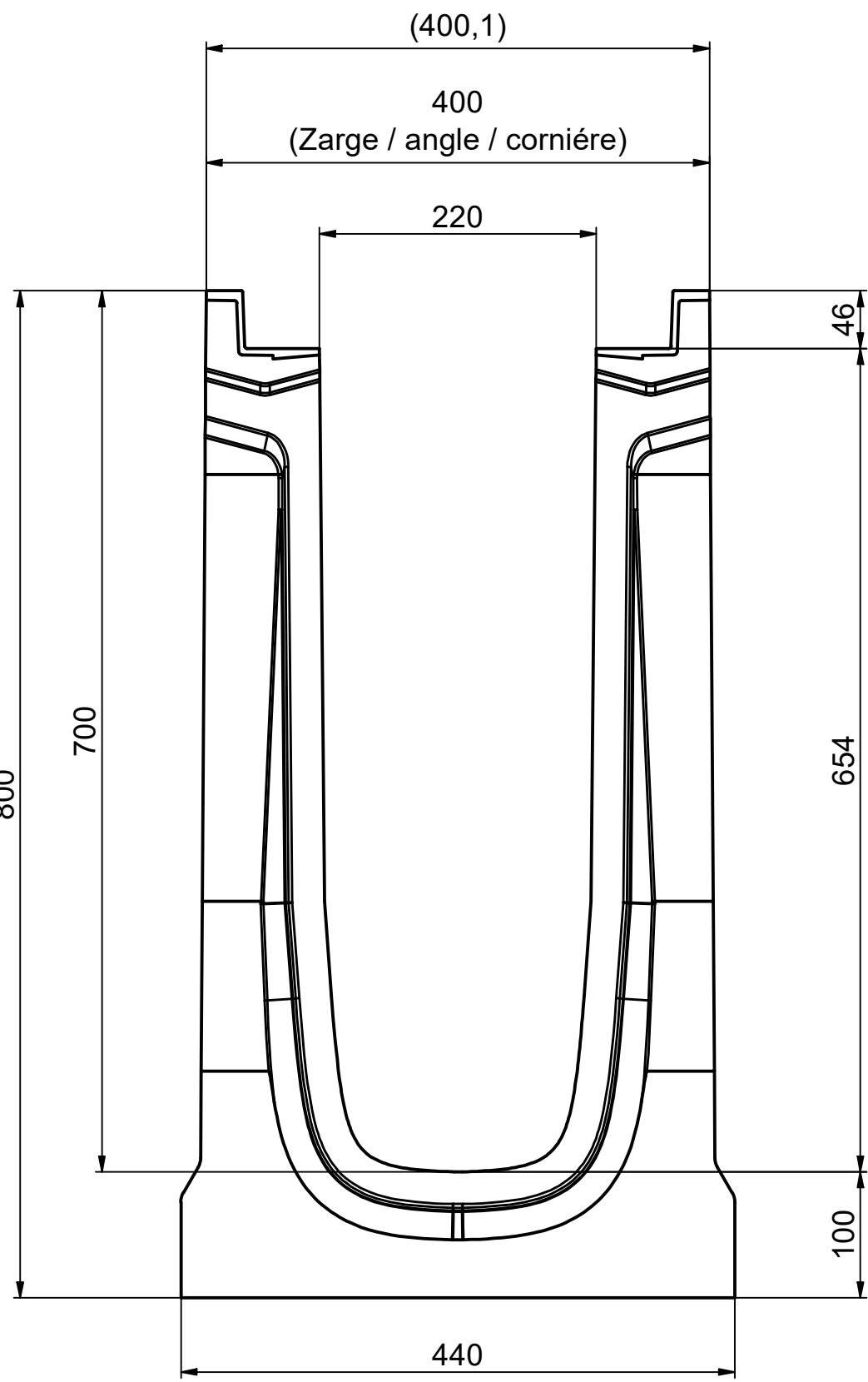
Ansicht Nut / view groove / vue rainure
