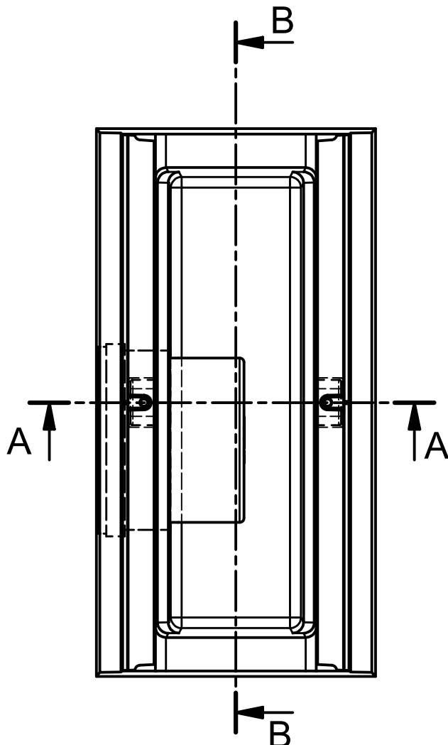
Draufsicht (ohne Schlammemeier) / top view (without silt bucket) / vue de dessus (représenté sans panier décanteur)
