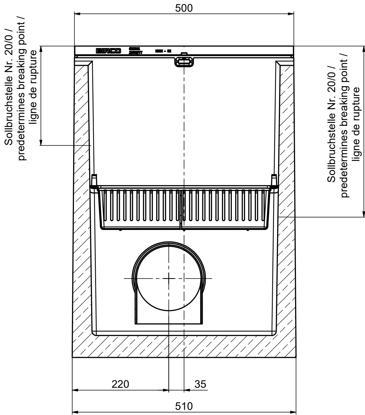
Schnitt / section / coupe B-B
