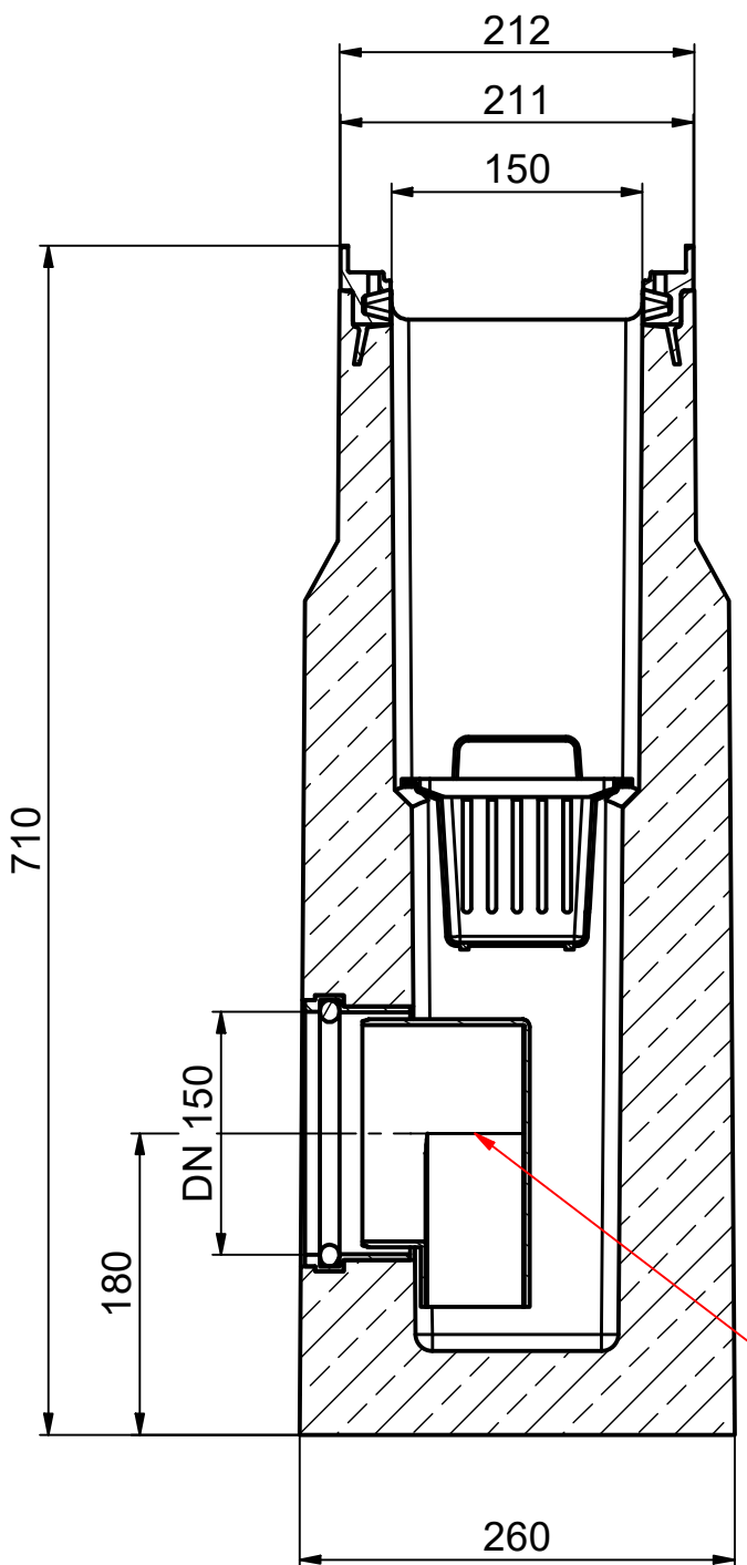
Schnitt / section / coupe A-A
