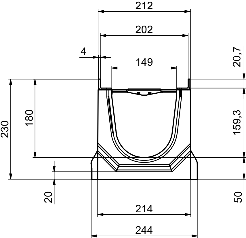
Ansicht Feder / view tongue / vue languette
