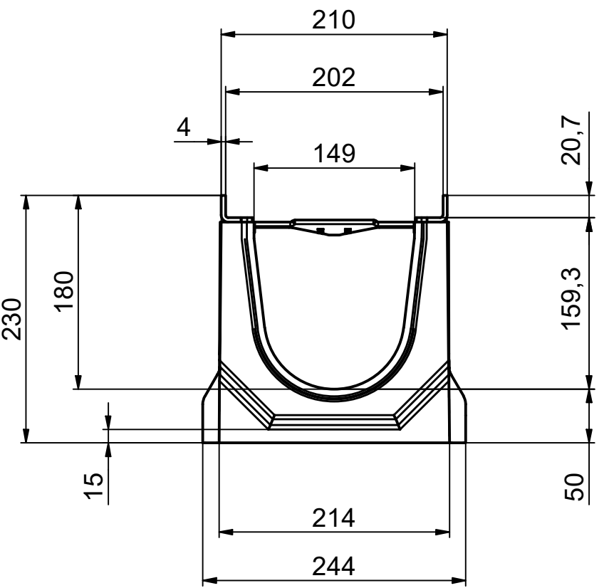
Ansicht Nut / view groove / vue rainure
