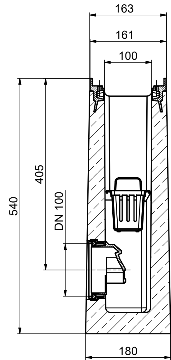
Schnitt / section / coupe A-A
