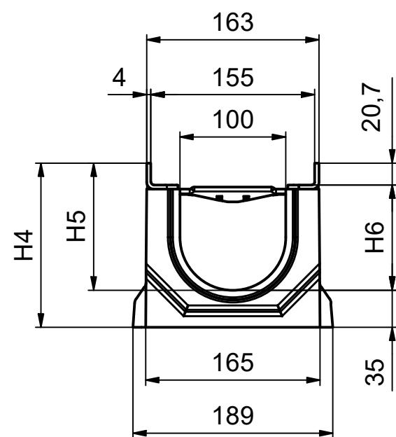
Ansicht Feder / view tongue / vue languette
