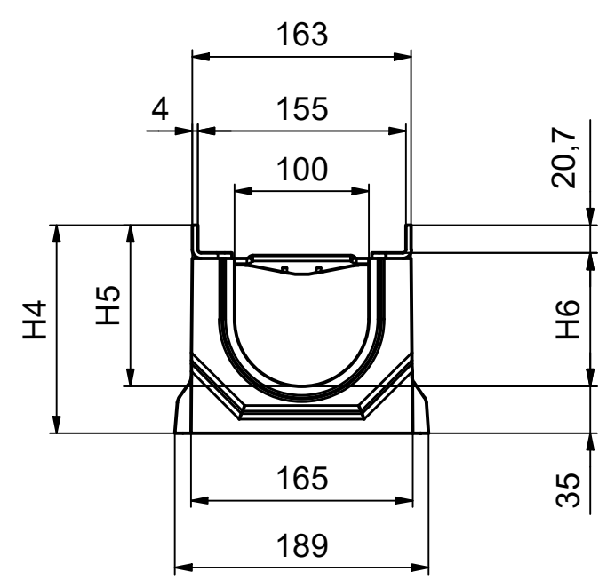
Ansicht Feder / view tongue / vue languette
