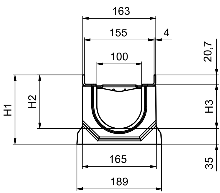
Ansicht Nut/ view groove / vue rainure
