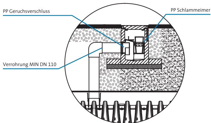
Entlüftungsvariante mit BIRCOsir Punktentwässerung 40x40
