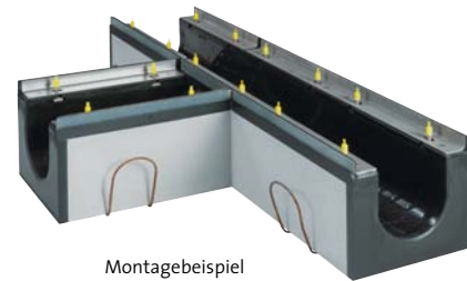
Montagebeispiel
