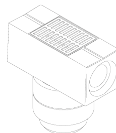
Caniveau avec sortie verticale longueur : 1,0 m
